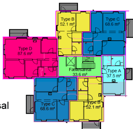
3. sal
