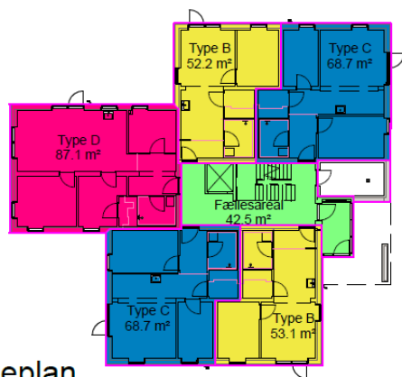
Stueplan
